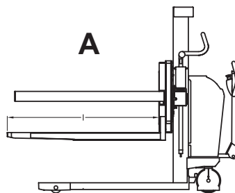
Περνοφόρο με πλευρικώς ανατρεπόμενα πιρούνια.
