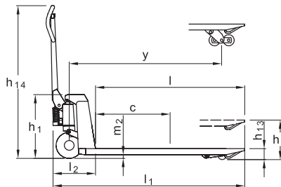
RF-PLUS - για τη βιομηχανία τροφίμων και τη φαρμακευτική βιομηχανία, όπου οι απαιτήσεις υγιεινής είναι υψηλές.
